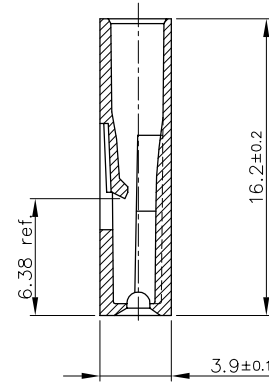
SECTION V-V
