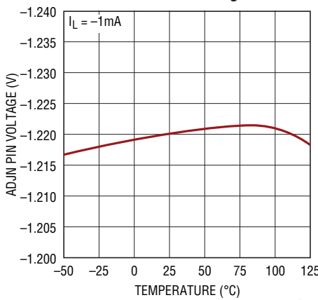
LT3032 ADJN Pin Voltage
