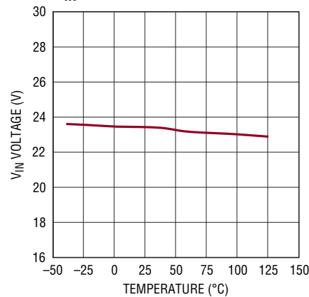
V_{\text{IN}} OVLO
