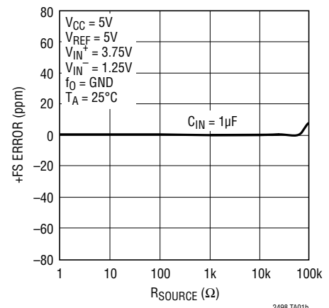
+FS Error vs R_{SOURCE}
