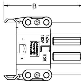
Stecker-Draufsicht
