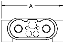
Stecker-Vorderansicht
