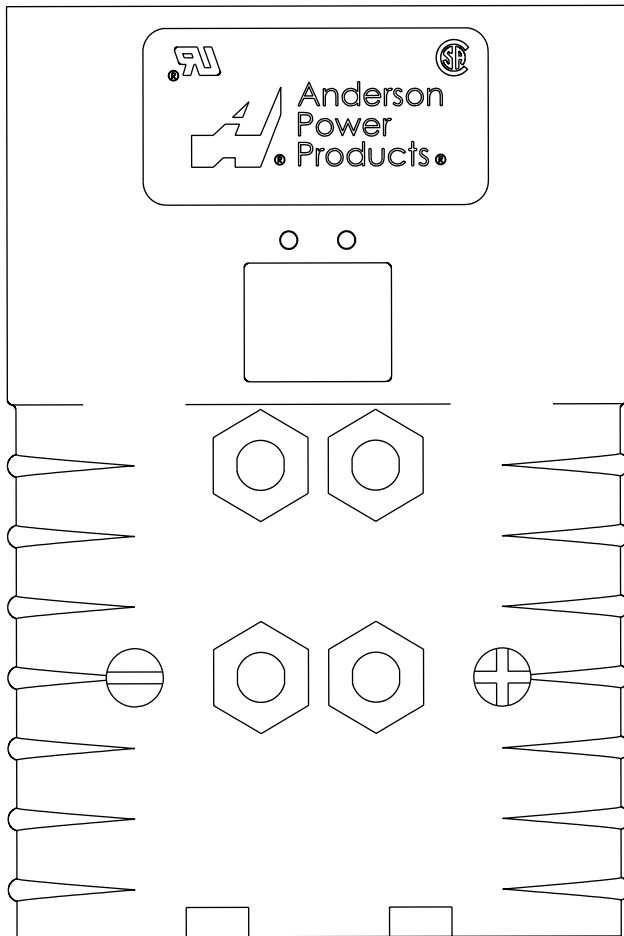
SBE® 320 / SBX® 350
