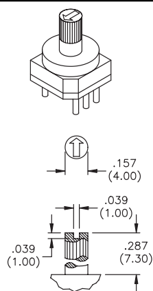
Spindle
