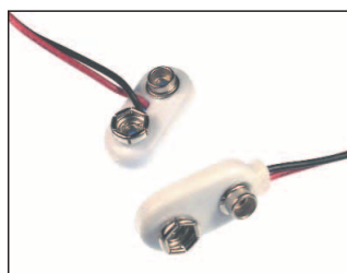
CCB-1 9V Battery connector. Cable length 220mm. Tough molded body. CCB-1A 'T' Type Cable length 220mm. CCB-1 (FC6830) CCB-1A (FC6831)
