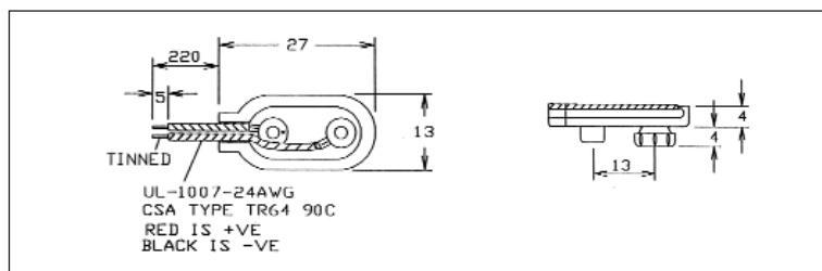
CCB-1 9V Battery connector. Cable length 220mm. Tough molded body. CCB-1A 'T' Type Cable length 220mm. CCB-1 (FC6830) CCB-1A (FC6831)
