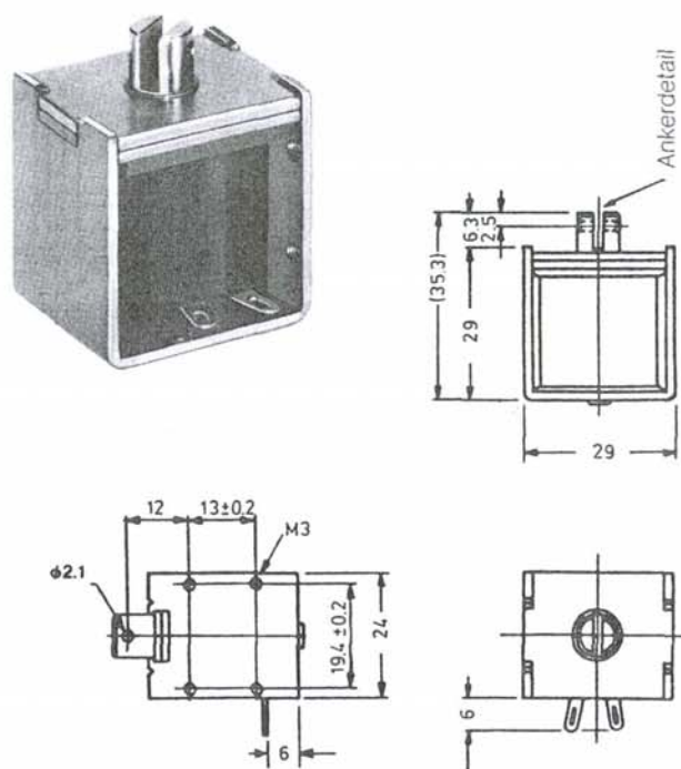
Ankerdetail
