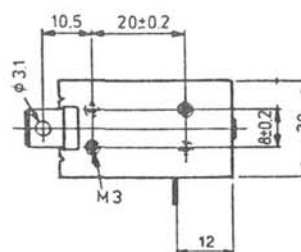
Ankerdetail
