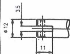
Ankerdetail
