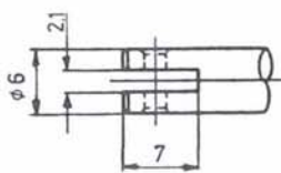
Ankerdetail
