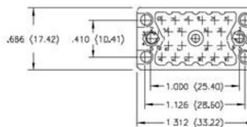
20 PIN RECEPTACLE
