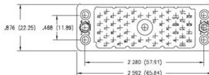
56 PIN RECEPTACLE
