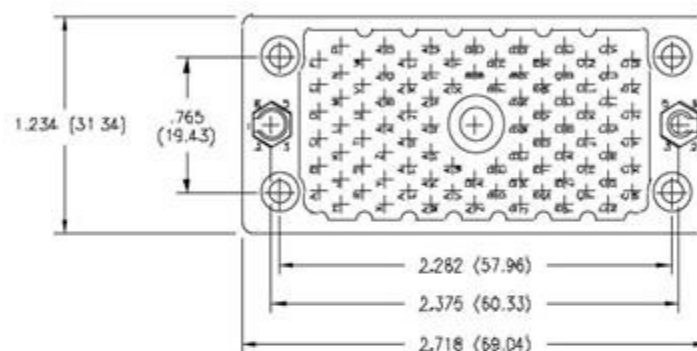
120 PIN RECEPTACLE
