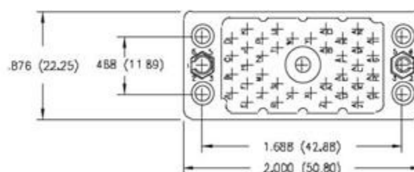
38 PIN RECEPTACLE
