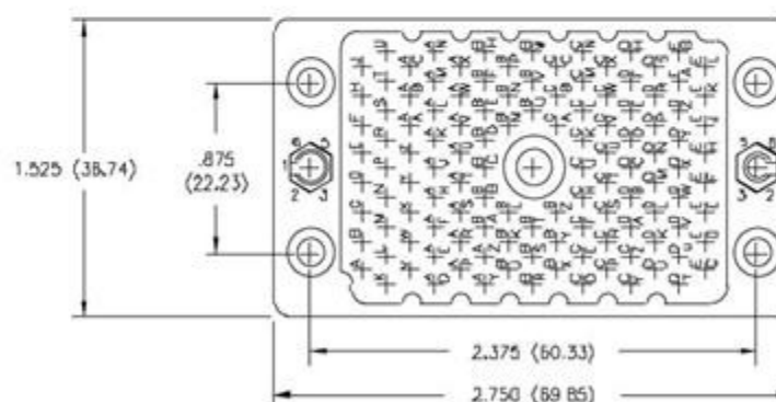
120 PIN RECEPTACLE
