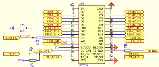
LCD
