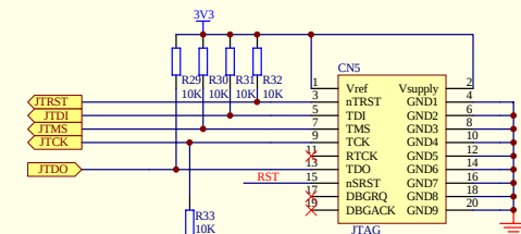
JTAG
