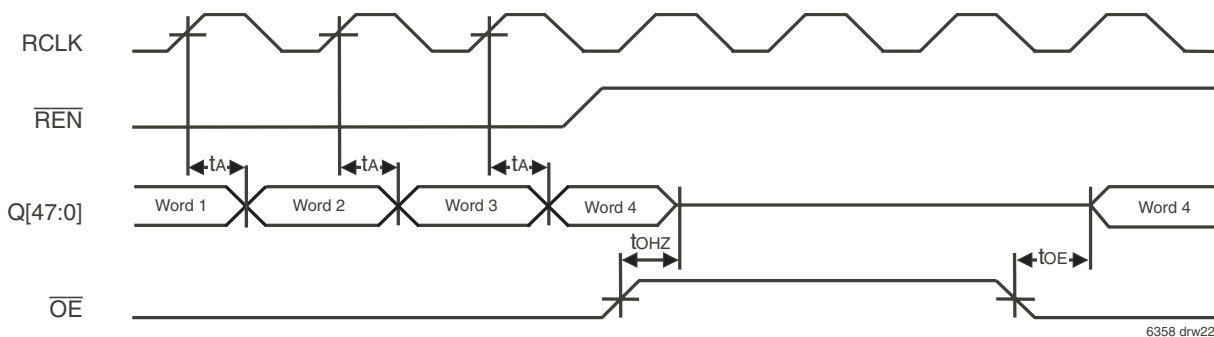
Figure 14. Output Enable
