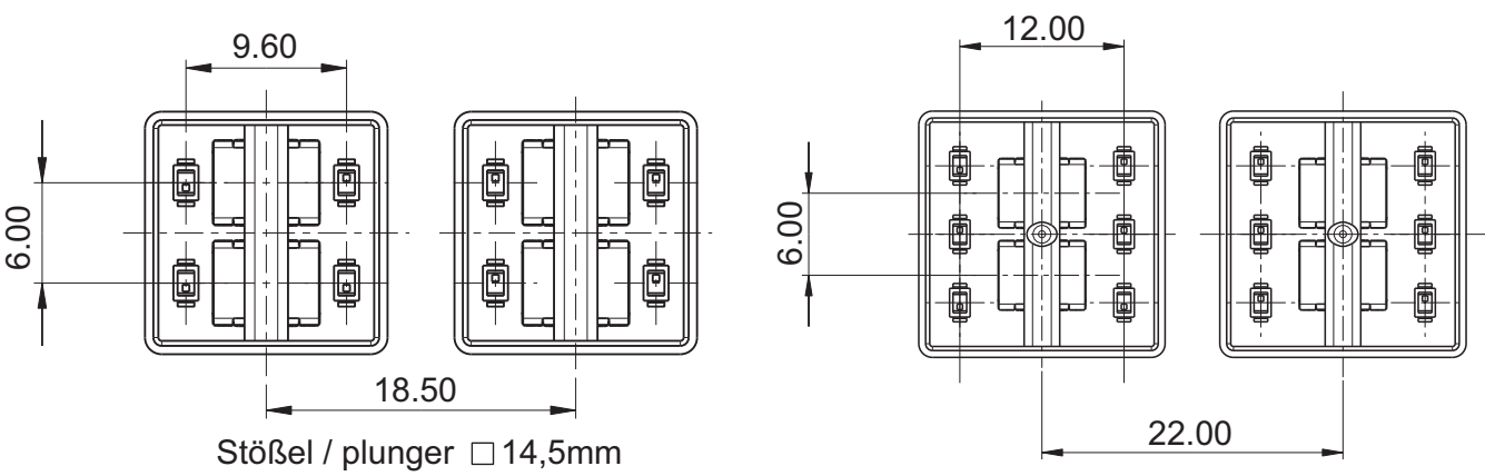
Plunger 14,5 x 14,5 mm
