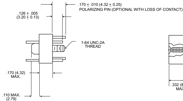
Receptacle
