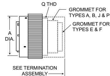
KPSE06/MS3126
