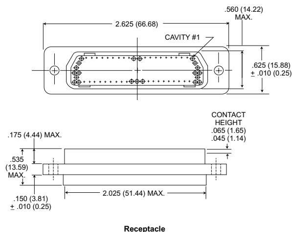
Receptacle
