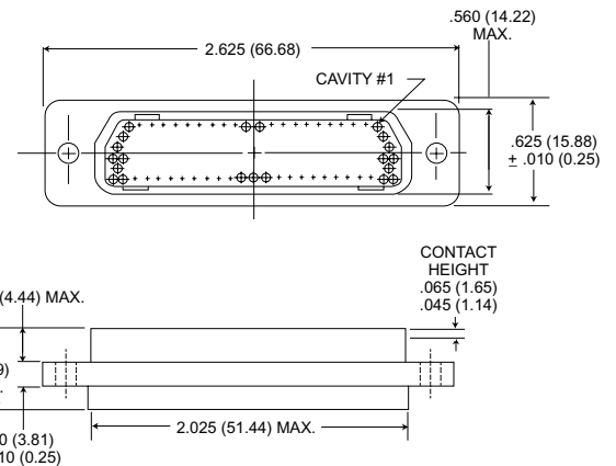
Receptacle
