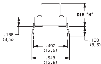
PTS125SM85 SPST
