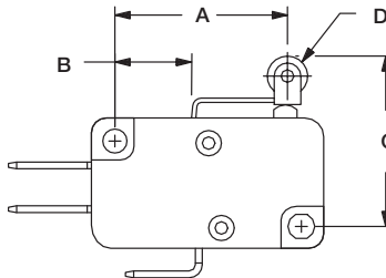
FIG. 1 Lever Roller
