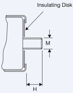
ALS35 Stud Mounting
