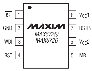
SOT23-8
