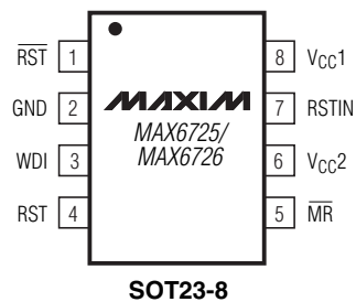
SOT23-8
