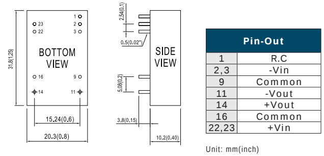
▲ RDDW08 1.25" x 0.8" x 0.40"
