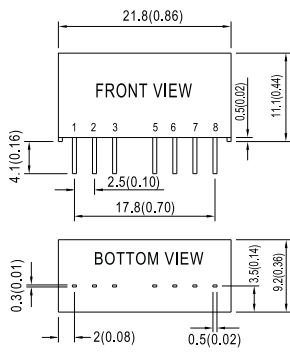
▲ SPBW03 0.86" x 0.36" x 0.44"
