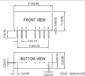
▲ SPB03 0.86" x 0.36" x 0.44"
