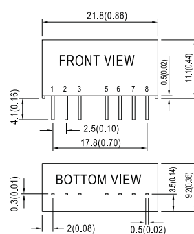
▲ SPBW06 0.86" x 0.36" x 0.44"
