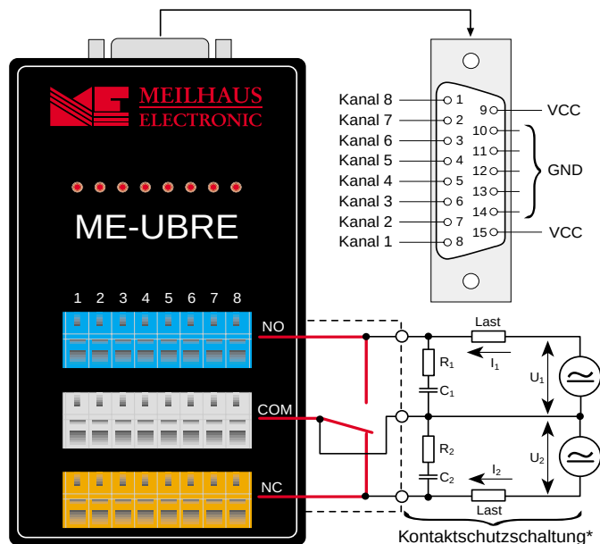
Abb. 1: Anschlußbelegung/Kontaktschutzschaltung
