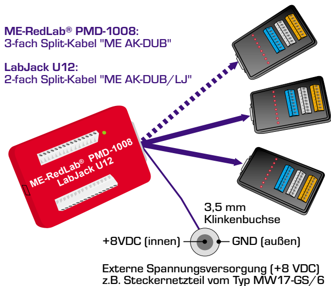
Abb. 2: Anschluß USB-Messboxen
