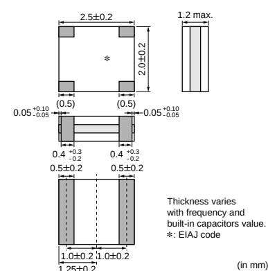
CSACW_X 20.00-70.00MHz
