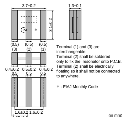
CSACV_X_Q 14.70-70.00MHz
