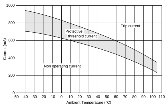
PTGLCSAS2R2K4B51B0
