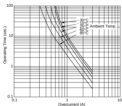
PTGL7SAS3R3K3B51B0
