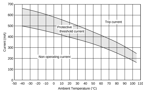
PTGL7SAS3R3K3B51B0
