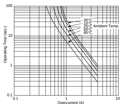
PTGL9SAS2R2K3B51B0
