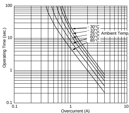
PTGL9SAS3R3K4B51B0
