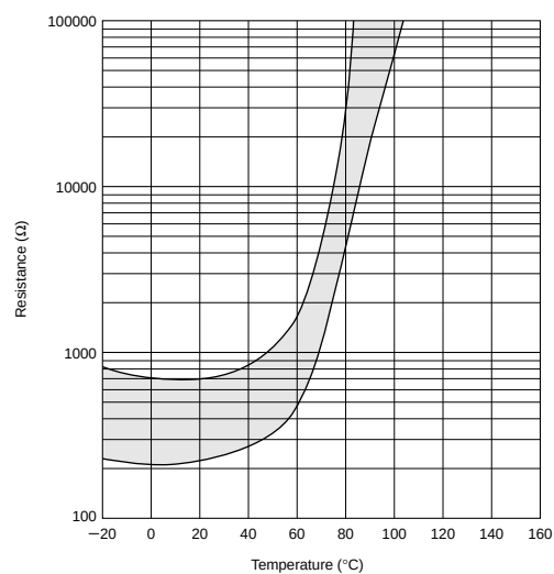
PRF18BF471QS2RB
