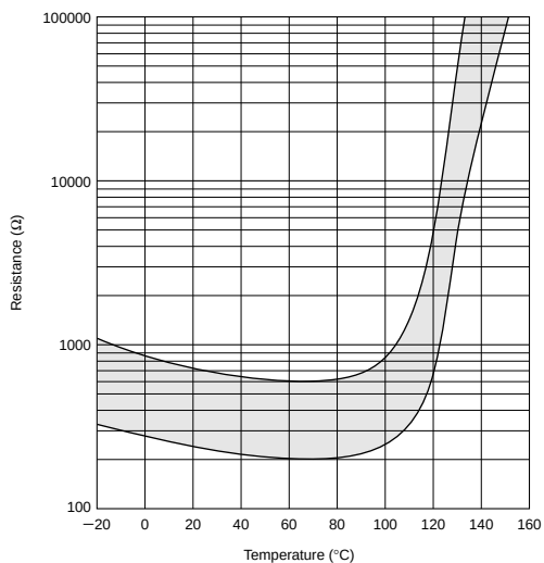
PRF18BA471QS2RB
