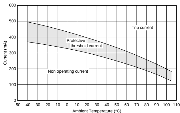
PTGL7SAS5R6K4B51B0
