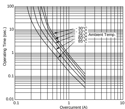
PTGL4SAS100K2B51B0
