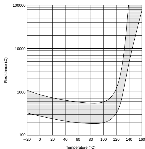
PRF18AR471QS2RB
