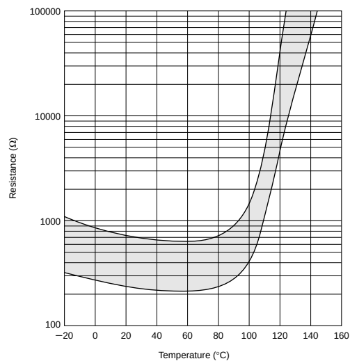
PRF18BB471QS2RB
