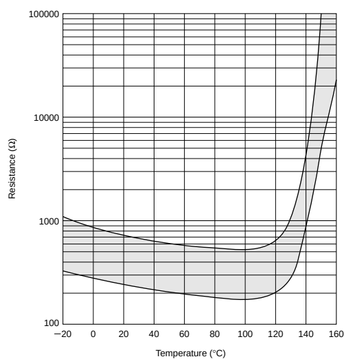
PRF18AS471QS2RB
