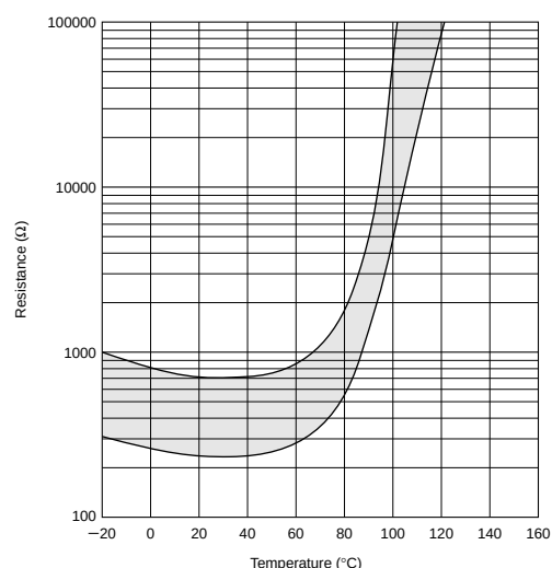
PRF18BD471QS2RB
