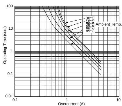
PTGL7SAS2R7K2B51B0
