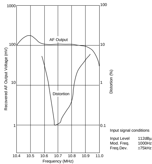
CDALF10M7GA048-B0
