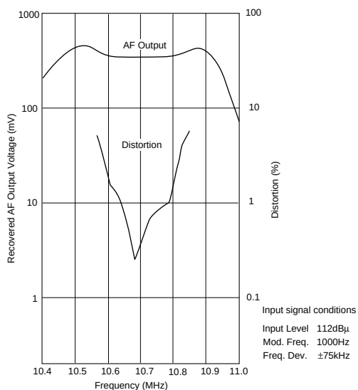
CDALF10M7GA046-B0
