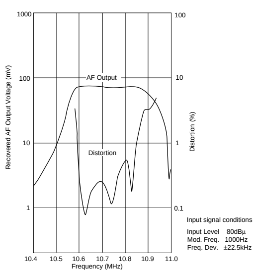
CDALF10M7GA018-B0
