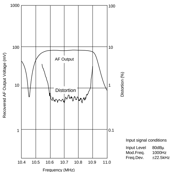
CDALF10M7GA092-B0
