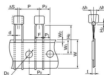
Taping Dimensions
