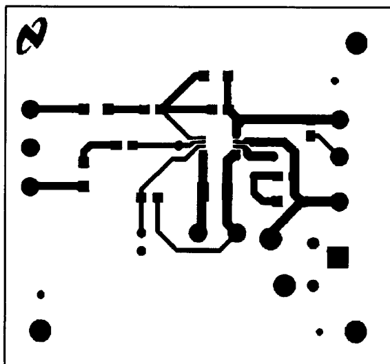
Top Layer
