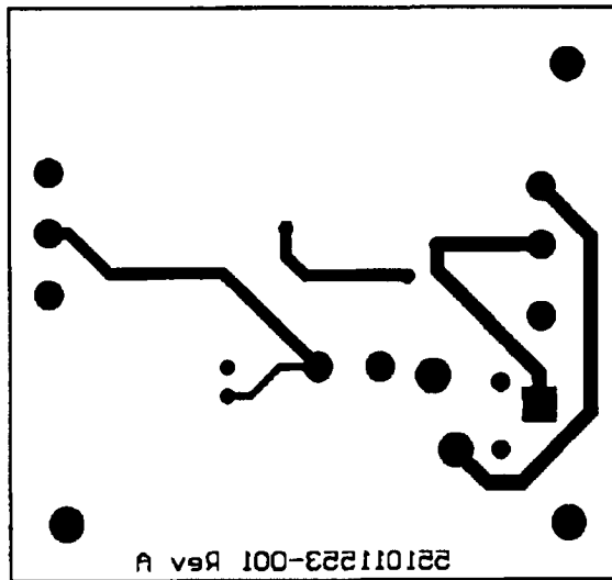
Bottom Layer
