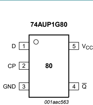
Fig. 4. Pin configuration SOT353-1 (TSSOP5)
