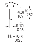
Straight PC (W03)
