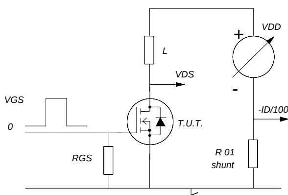
Fig.18. Avalanche energy test circuit. W_{DSS} = 0.5 \cdot L I_D^2 \cdot BV_{DSS} / (BV_{DSS} - V_{DD})
