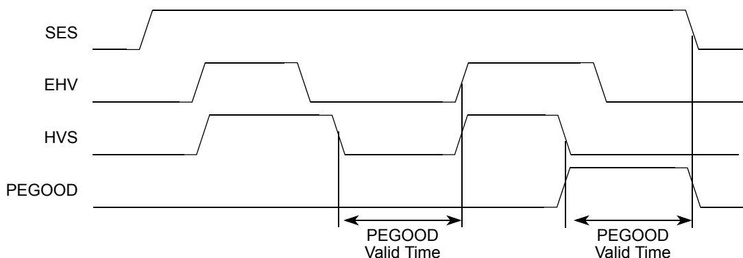
Figure 21-5. PEGOOD Valid Time
