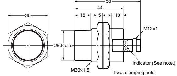
E2A-M30KN20-M1-□□/E2A-S30KN20-M1-□
