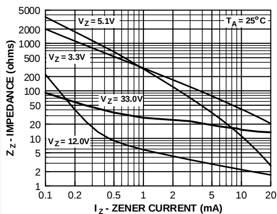
Zener Current vs. Zener Impedance
