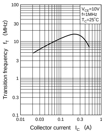
f_T - I_C
