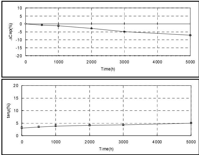
EEUEB2G100 (400V10 \mu F, \phi 16X16.5L)
