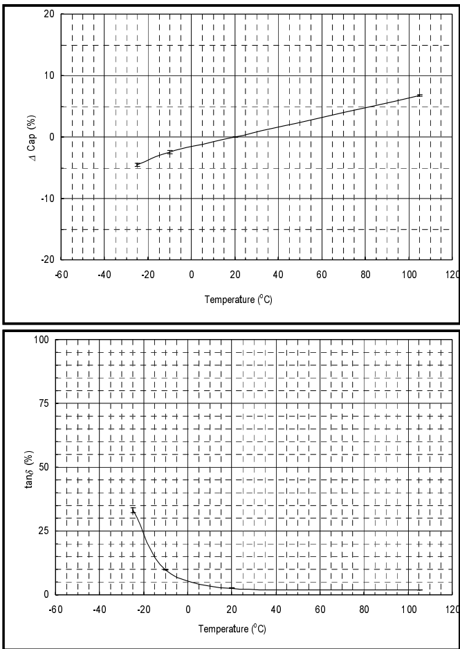
EEUEB2G100 (400V10 \mu F, \phi 16x16.5L)
