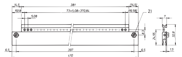
2) Press-in insert M4
