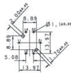
Lochbild Leiterplatte, Bauteilseite
