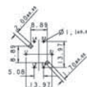
Lochbild Leiterplatte, Bauteilseite
