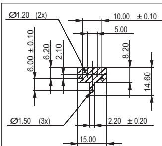
Sicht auf Bestückungsseite
