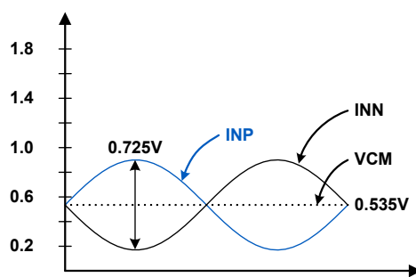
Figure 28. Analog Input Range
