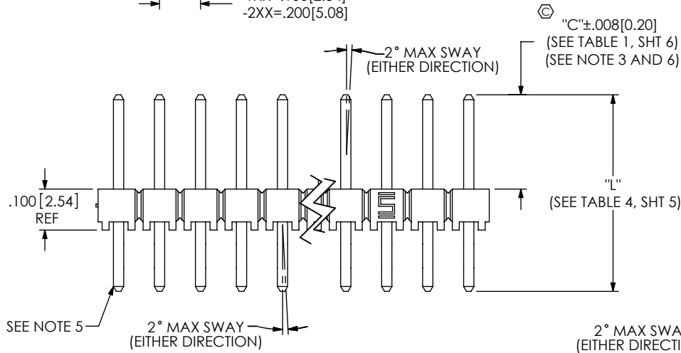
FIG 1 (TSW-1XX-XX-XX-S SHOWN)
