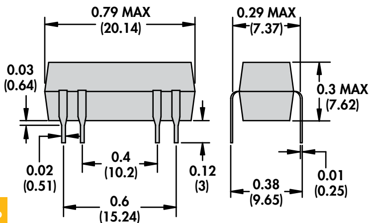
172DIP SPDT
