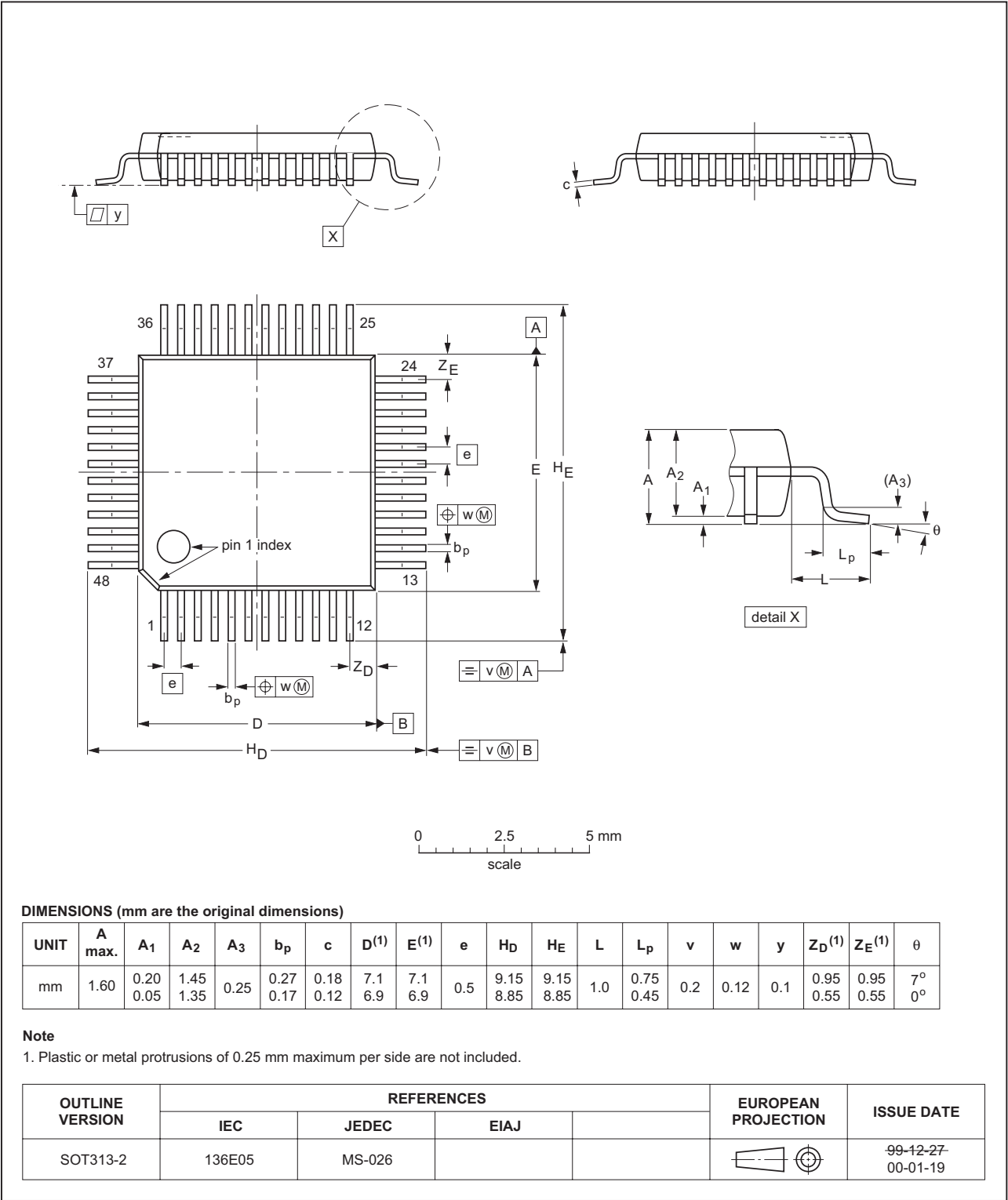
Fig 33. LQFP48 (SOT313-2).
