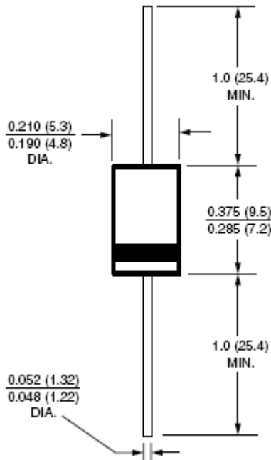
DO-201AD
