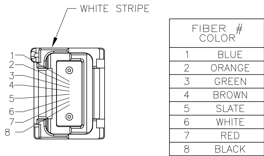
VIEW A-A
