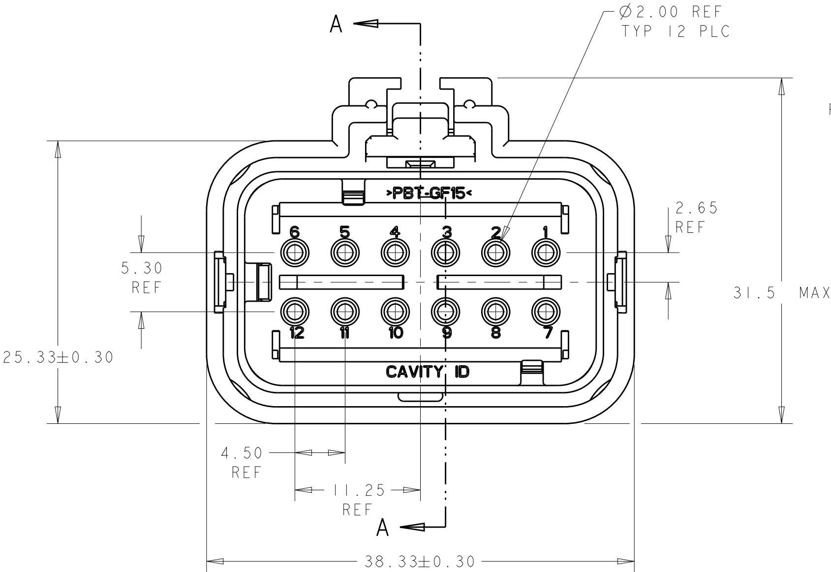
776437-1 SHOWN
