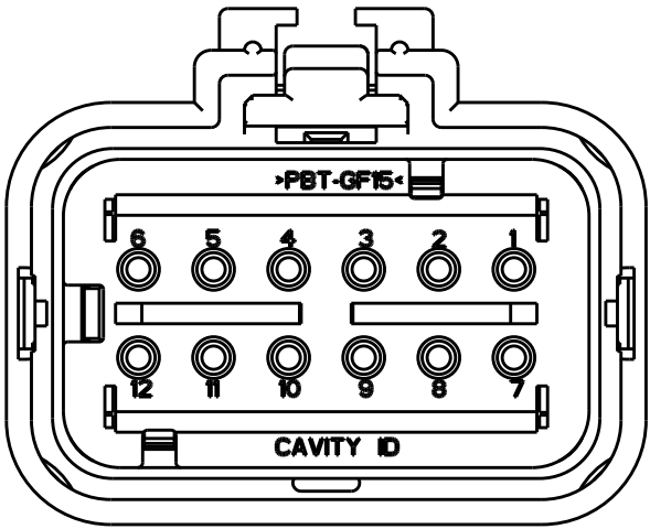
776437-2 SCALE 2:1
