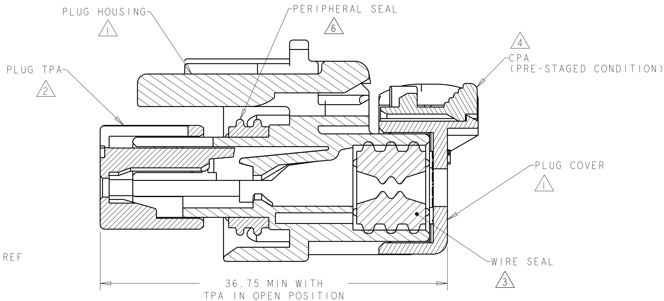
SECTION A-A
