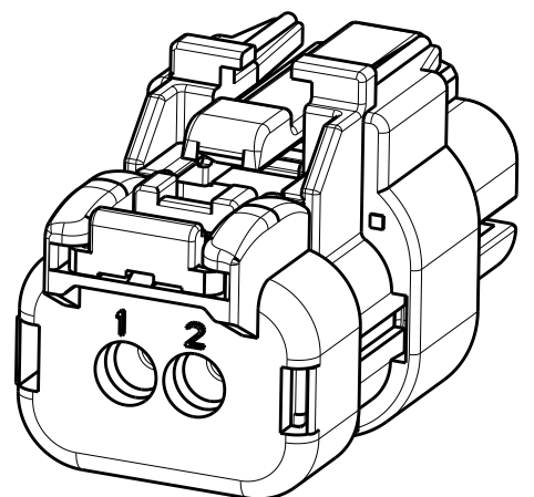
SCALE 2:1
