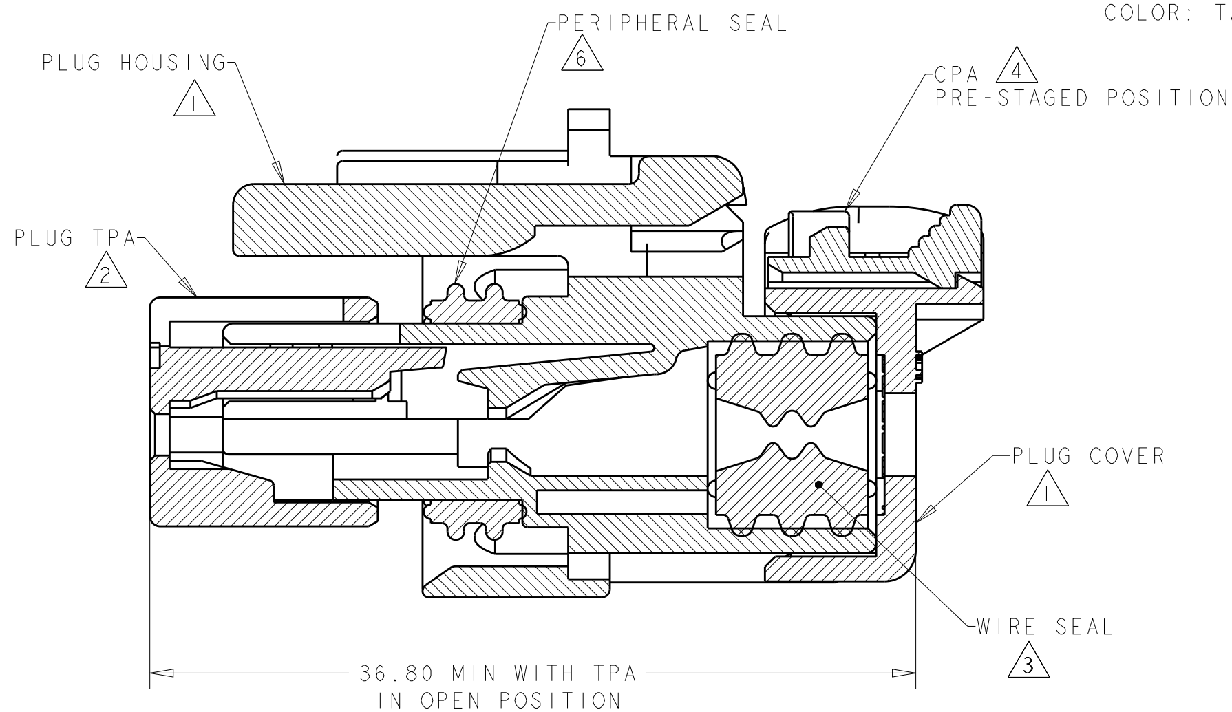
SECTION A-A
