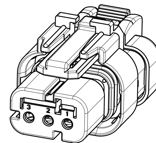
SCALE 2:1
