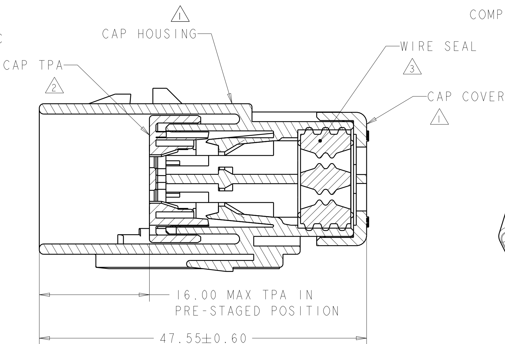
SECTION A-A
