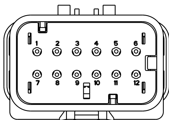
776539-4 SCALE 2:1
