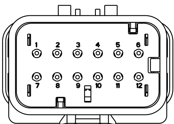
776539-3 SCALE 2:1
