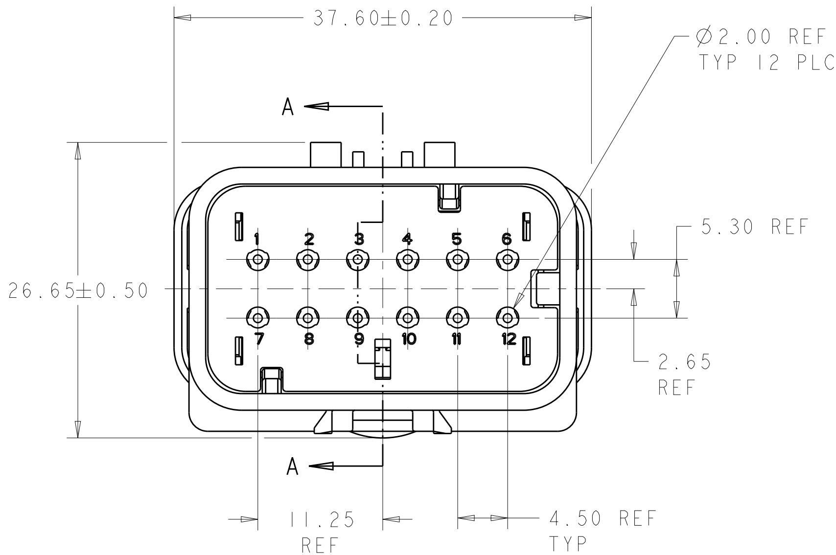
776539-1 SHOWN
