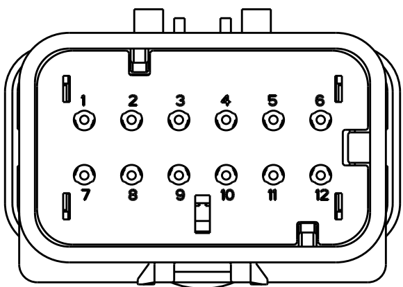
776539-2 SCALE 2:1
