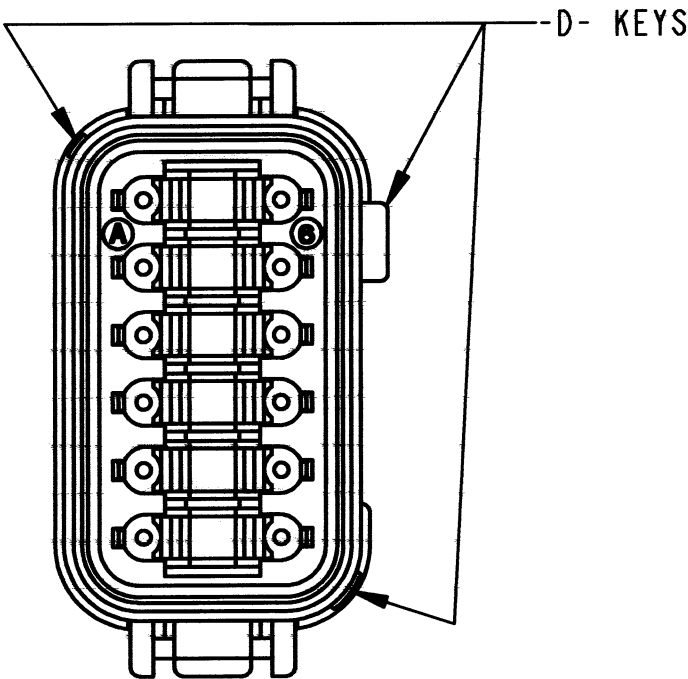
DT06-12SD-CE05 KEY ARR. -D- COLOR: BROWN
