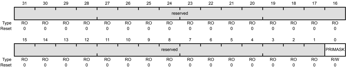
Priority Mask Register (PRIMASK)
